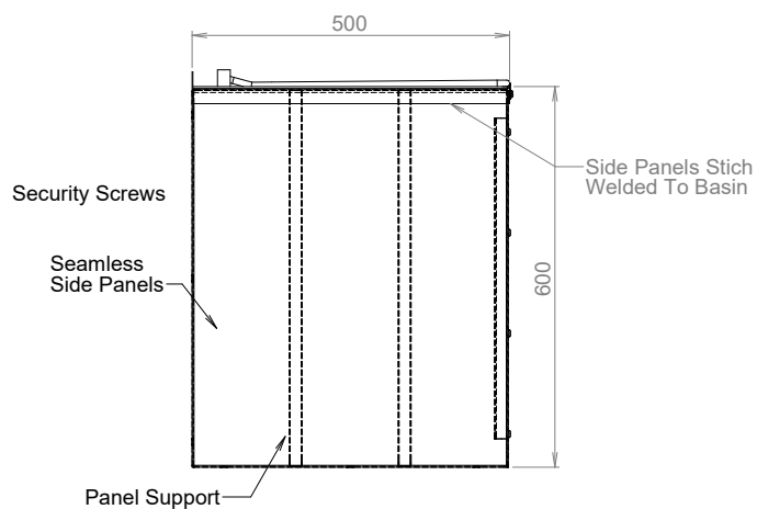
MODEL CS-SEC Side View
