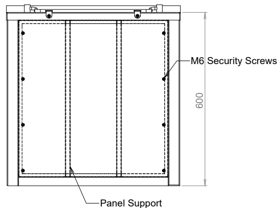
MODEL CS-SEC Rear View
